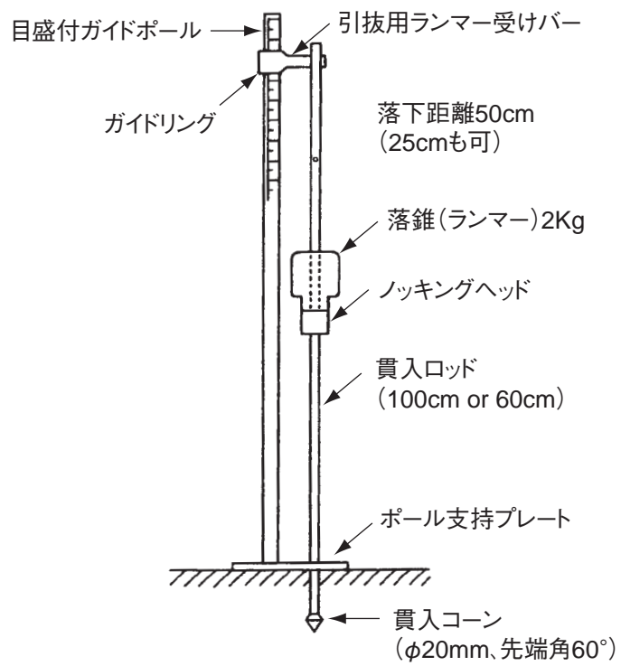
図3 長谷川式土壌貫入計
